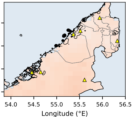
c ERA5-Land Tmin
