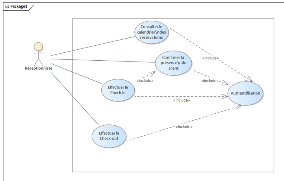
FIGURE 2.2 – Diagramme de cas d'utilisation — Réceptionniste
