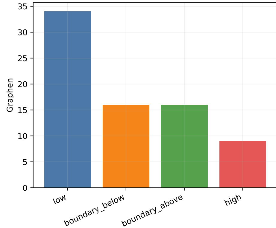
Ausgewählte Wahrscheinlichkeitsbereiche
