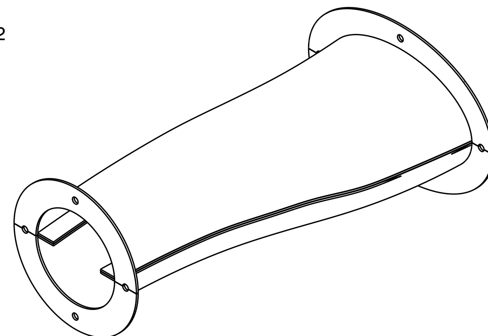
Vue isométrique Echelle : 1:3
