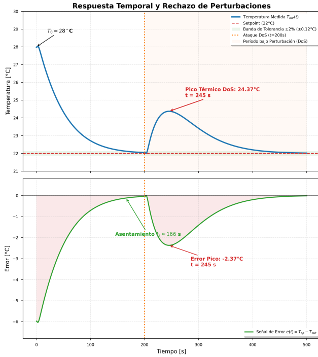
Figura 10. Respuesta completa del sistema. Superposición del seguimiento al escalón de referencia ( 28 \rightarrow 22^\circ\text{C} ) y el rechazo del ataque DoS inyectado en t = 200 s. En ambas fases el error en régimen permanente es nulo.
