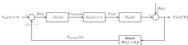
Figura 7. Diagrama de bloques simplificado para el análisis de perturbación ( R(s) = 0 ). La referencia se anula y la perturbación D(s) se suma después de la planta con signo positivo, modelando el aumento aditivo de temperatura provocado por el ataque DoS.
