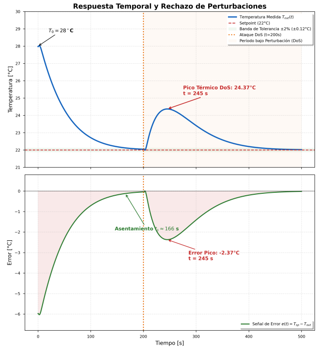
Figura 10. Respuesta completa del sistema. Superposición del seguimiento al escalón de referencia ( 28 \rightarrow 22^{\circ}\text{C} ) y el rechazo del ataque DoS inyectado en t = 200 s. En ambas fases el error en régimen permanente es nulo.
