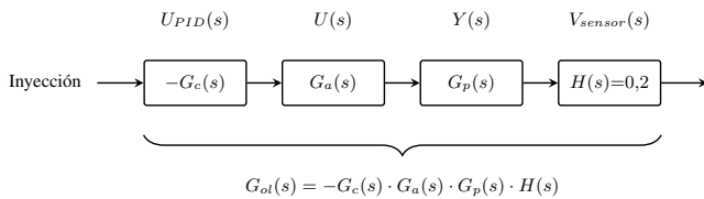
Figura 3. Concepto de ganancia de lazo abierto G_{ol}(s) . Al abrir el lazo antes del comparador e inyectar una señal de prueba, se recorre en serie el controlador, el actuador, la planta y el sensor. El producto de estas cuatro transferencias define G_{ol}(s) .
