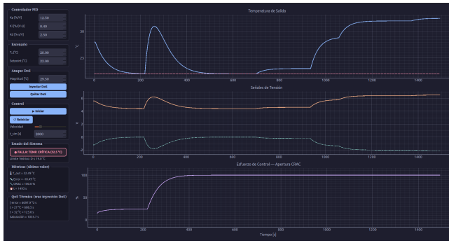
Figura 12. Captura del simulador ante un DoS extremo de D = 29,5^\circ\text{C} . La potencia de enfriamiento resulta insuficiente, provocando que la temperatura del aire supere el límite crítico absoluto de seguridad de 32^\circ\text{C} .
