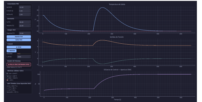
Figura 11. Captura del simulador para una perturbación límite de D = 19^\circ\text{C} . El sistema estabiliza la temperatura en 22^\circ\text{C} , pero exige el 100 % del esfuerzo de control de los ventiladores, de modo que el simulador declara una falla por capacidad tras 30 s continuos de saturación.
