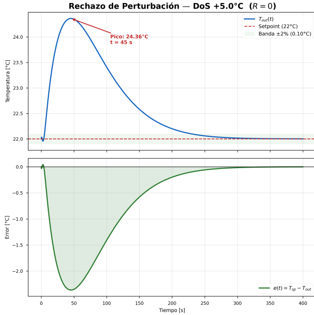
Figura 8. Rechazo de perturbación ( R = 0 ). Simulación del efecto de un ataque DoS de +5 °C. El gráfico superior muestra la temperatura de salida T_{out}(t) (curva azul sólida), la cual parte del setpoint de 22 °C (línea discontinua roja), alcanza un pico máximo de 24,36 °C a los t = 45 s debido a la inercia térmica y regresa progresivamente a la banda de tolerancia de \pm 2 % (franja sombreada verde). El gráfico inferior muestra la señal de error de regulación e(t) (curva verde sólida); el área sombreada bajo dicha curva representa gráficamente la Severidad de la Excursión Térmica (TES), la cual es anulada en estado estacionario gracias a la acción integral.
