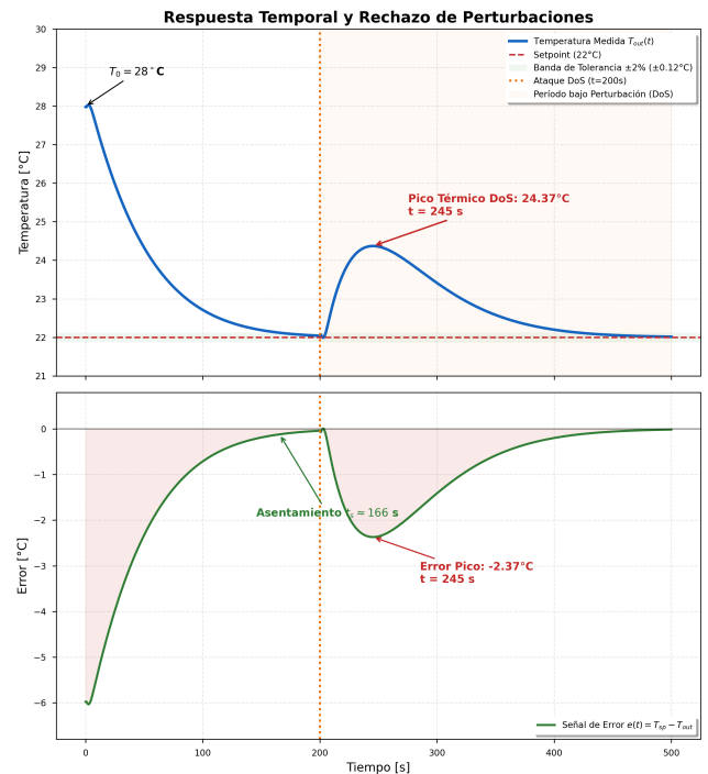
Figura 10. Respuesta completa del sistema. Superposición del seguimiento al escalón de referencia ( 28 \rightarrow 22^{\circ}\text{C} ) y el rechazo del ataque DoS inyectado en t = 200 \text{ s} . En ambas fases el error en régimen permanente es nulo.
