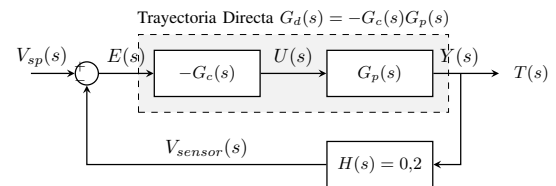
Figura 4. Diagrama de bloques simplificado del lazo de control, destacando la Trayectoria Directa G_d(s) con la inversión de signo incorporada y la realimentación a través del sensor H(s) para obtener G_{ol}(s) = G_d(s)H(s) .
