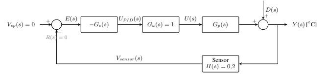
Figura 7. Diagrama de bloques simplificado para el análisis de perturbación ( R(s) = 0 ). La referencia se anula y la perturbación D(s) se suma después de la planta con signo positivo, modelando el aumento aditivo de temperatura provocado por el ataque DoS.
