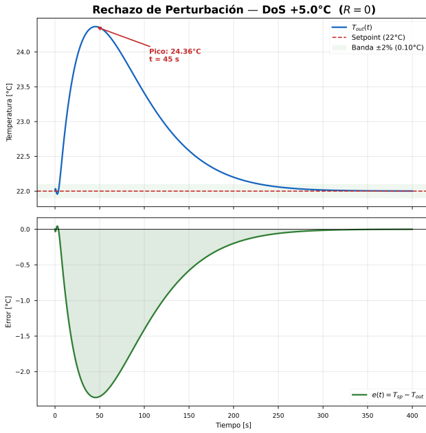
Figura 8. Rechazo de perturbación. Partiendo del estado estacionario en 22 °C, se inyecta un escalón de +5 °C filtrado por la dinámica FOPTD del pasillo frío. La temperatura asciende suavemente hasta un pico de 24,36 °C y es llevada de regreso al setpoint en aproximadamente 229 s.
