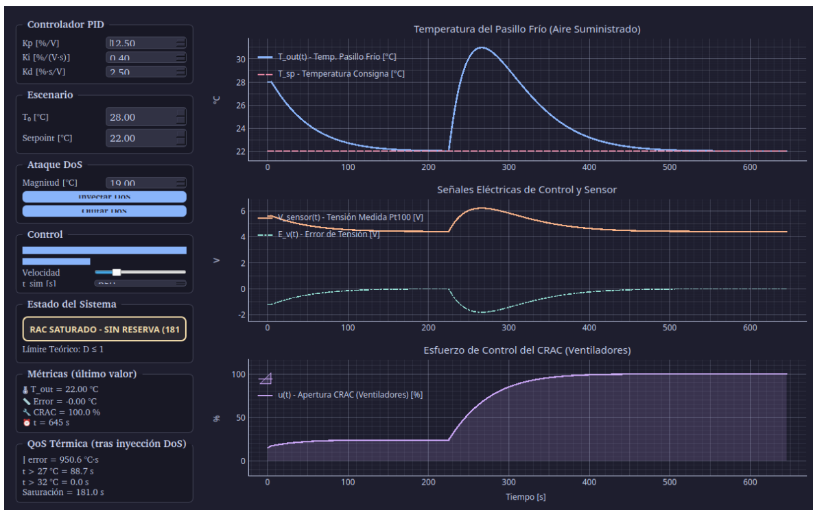
Figura 11. Captura del simulador para una perturbación límite de D = 19^\circ\text{C} . El sistema estabiliza la temperatura en 22^\circ\text{C} , pero exige el 100 % del esfuerzo de control de los ventiladores, de modo que el simulador declara una falla por capacidad tras 30 s continuos de saturación.
