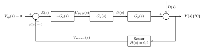
Figura 7. Diagrama de bloques simplificado para el análisis de perturbación ( R(s) = 0 ). La referencia se anula y la perturbación D(s) se suma después de la planta con signo positivo, modelando el aumento aditivo de temperatura provocado por el ataque DoS.
