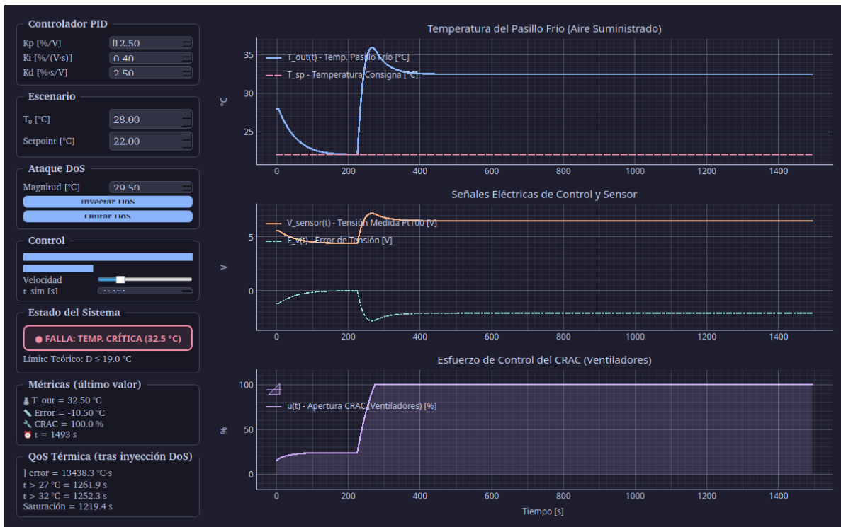
Figura 12. Captura del simulador ante un DoS extremo de D = 29,5\text{ }^{\circ}\text{C} . La potencia de enfriamiento resulta insuficiente, provocando que la temperatura del aire supere el límite crítico absoluto de seguridad de 32\text{ }^{\circ}\text{C} .
