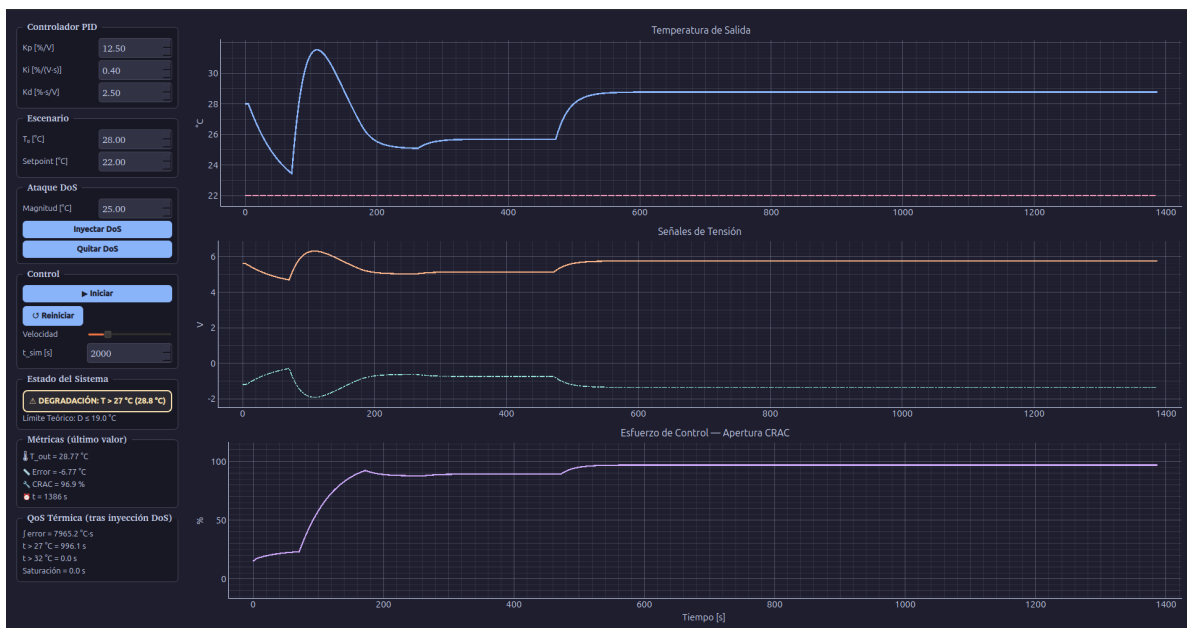
Figura 13. Diagnóstico experimental de la saturación prematura. Debido a un límite de sujeción integral de \pm 200 , la acción integral se bloqueaba limitando el esfuerzo del CRAC al 96,9 % y dejando un desvío térmico permanente de -6,77\text{ }^{\circ}\text{C} .
