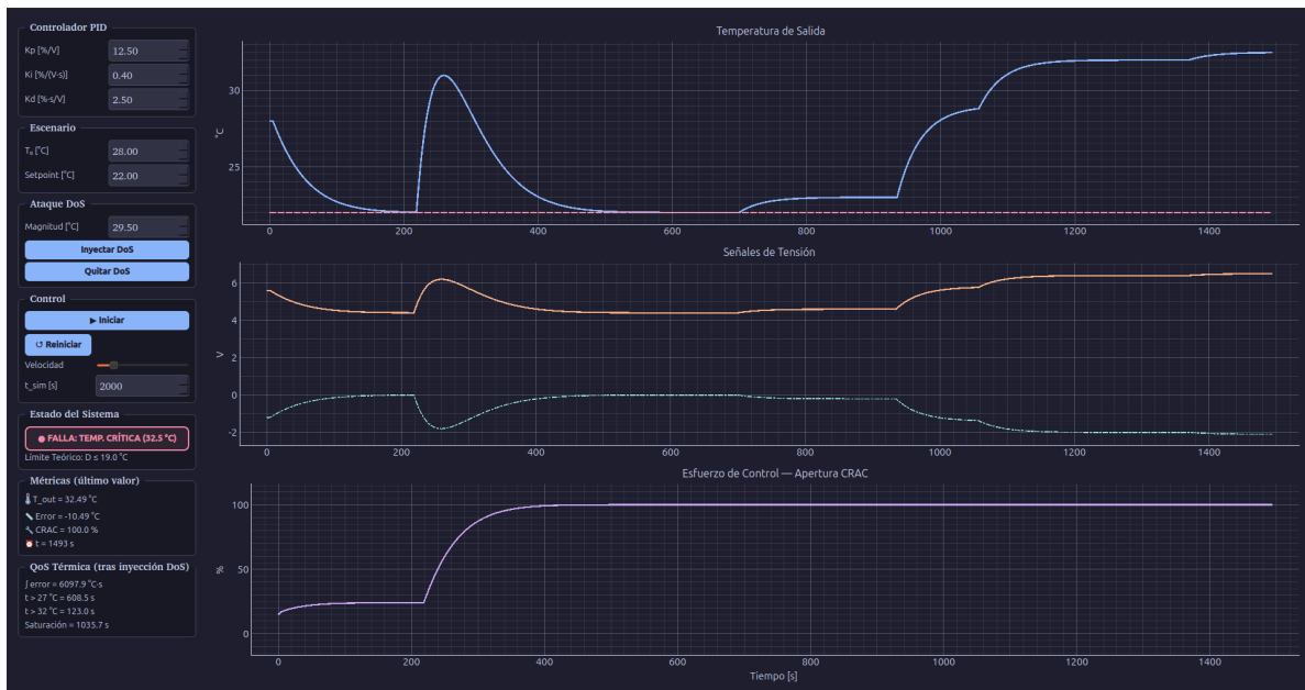
Figura 12. Captura del simulador ante un DoS extremo de D = 29,5\text{ }^{\circ}\text{C} . La potencia de enfriamiento resulta insuficiente, provocando que la temperatura del aire supere el límite crítico absoluto de seguridad de 32\text{ }^{\circ}\text{C} .
