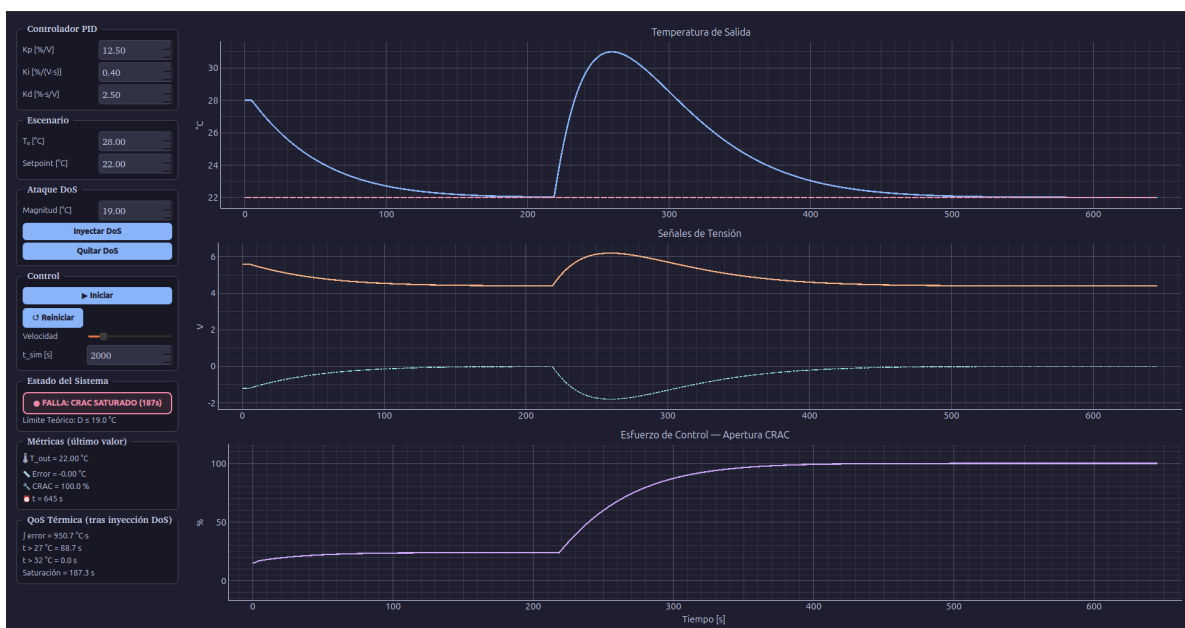
Figura 11. Captura del simulador para una perturbación límite de D = 19^\circ\text{C} . El sistema estabiliza la temperatura en 22^\circ\text{C} , pero exige el 100 % del esfuerzo de control de los ventiladores, de modo que el simulador declara una falla por capacidad tras 30 s continuos de saturación.
