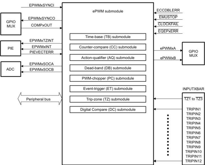
Figura 3.13: Diagrama de bloques y submódulos del periférico ePWM [34].
