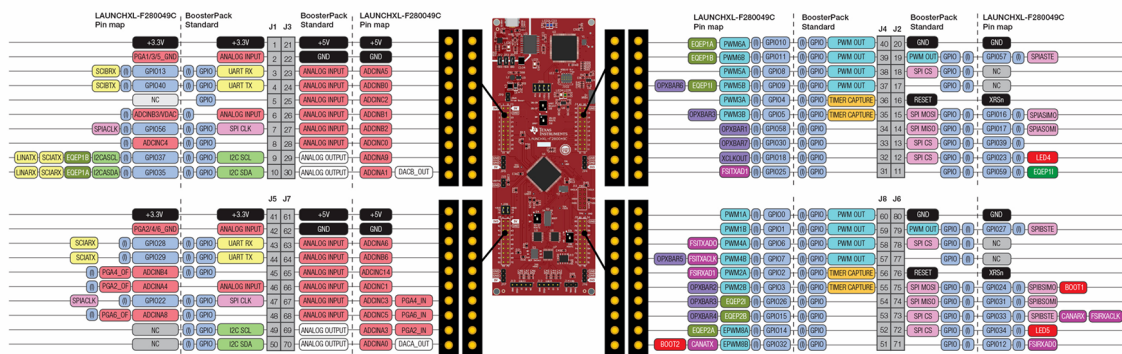
Figura 3.11: Mapa de pines y asignación de periféricos de la tarjeta LAUNCHXL-F280049C [33]
