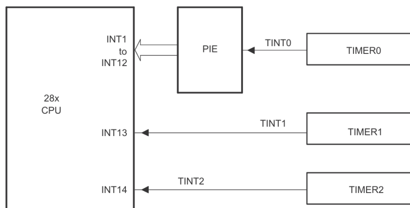
Figura 3.17: Rutas de las señales de interrupción asociadas a los TIMERS [34].
