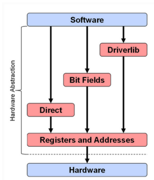
Figura 3.9: Niveles de abstracción para programar el microcontrolador [32]
