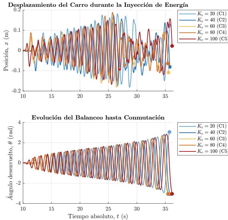
Figura 4.5: Desempeño de los controladores sobre la planta real
