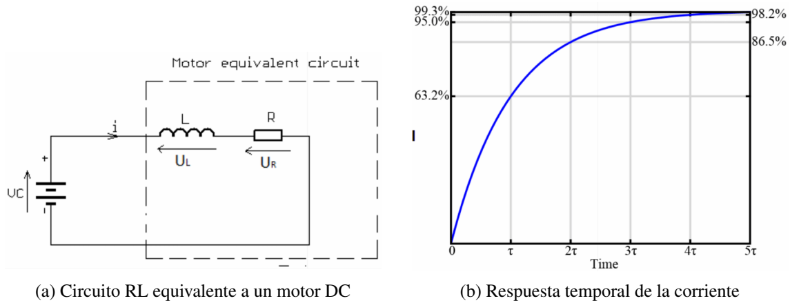
Figura 6.1: Circuito equivalente de un circuito motor DC y su dinámica ante entrada escalón [39]
