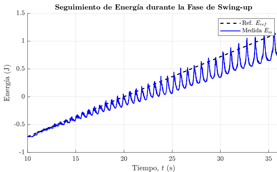
Figura 3.28: Referencia rampa y seguimiento por el control de energía
