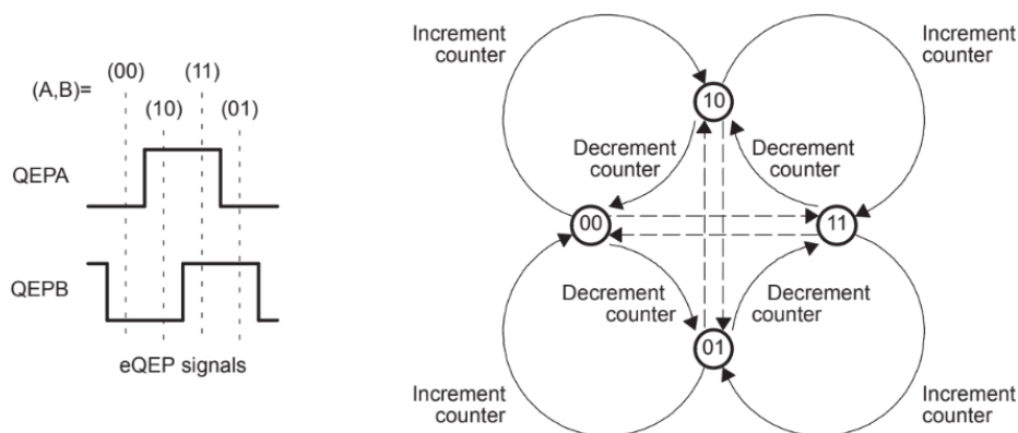
Figura 3.12: Máquina de estados, decodificación en cuadratura [34]
