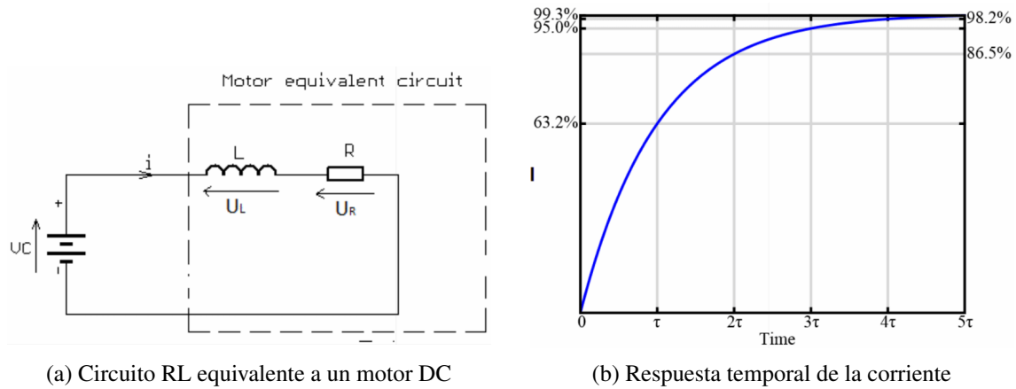
Figura 6.1: Circuito equivalente de un circuito motor DC y su dinámica ante entrada escalón [30]
