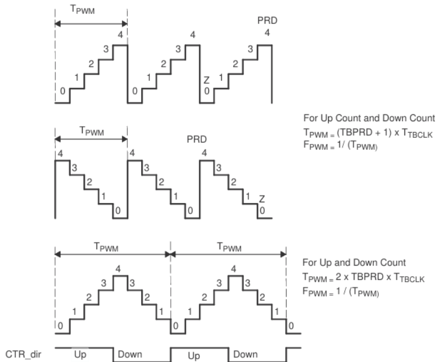
Figura 3.14: Modos de conteo del submódulo Time-base (TB) y ecuaciones de periodo [26].
