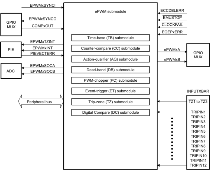
Figura 3.13: Diagrama de bloques y submódulos del periférico ePWM [26].
