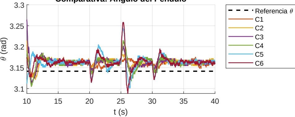
Comparativa: Ángulo del Péndulo
