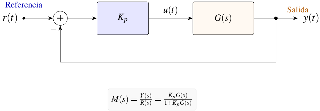
Figura 3.22: Control P para identificación en BC
