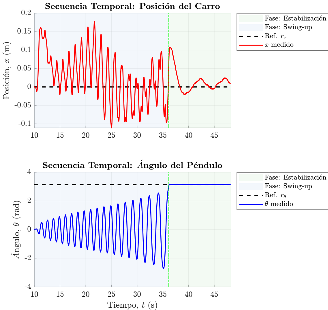
Figura 4.5: Control híbrido, conmutación entre Swing-up y control de posición
