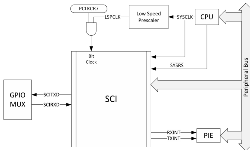
Figura 3.15: Diagrama de bloques y conexiones principales del periférico SCI [22]
