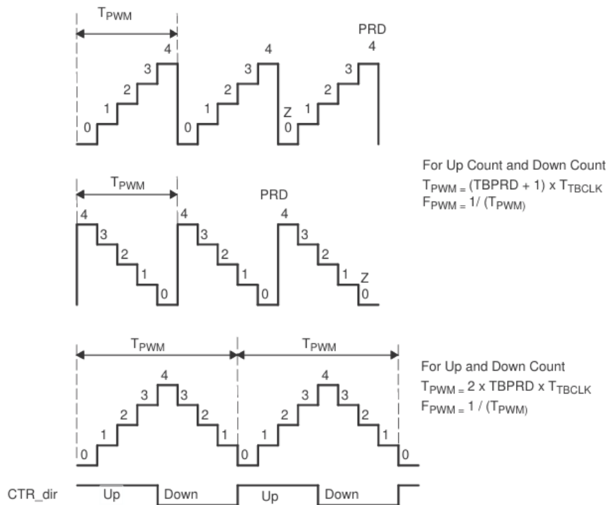
Figura 3.14: Modos de conteo del submódulo Time-base (TB) y ecuaciones de periodo [22].
