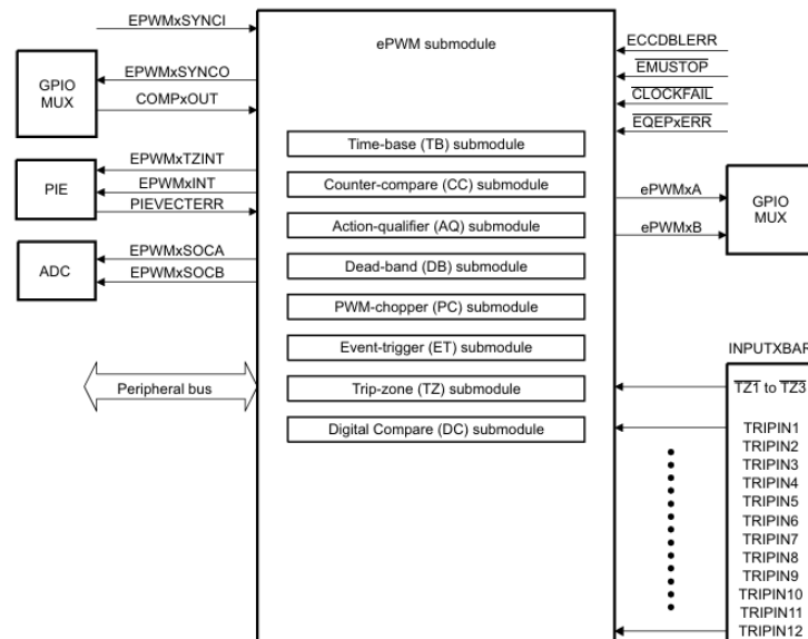
Figura 3.13: Diagrama de bloques y submódulos del periférico ePWM [22].
