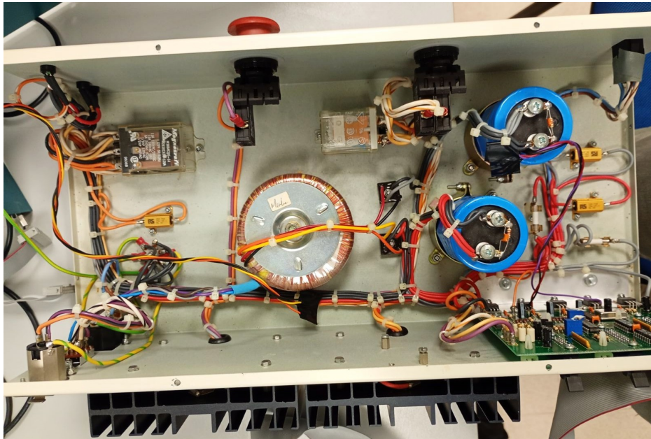
Figura 1.2: Controlador digital original
