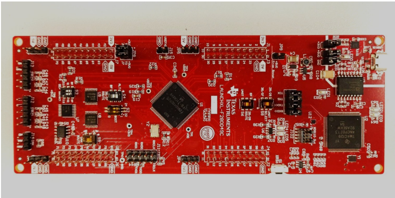
Figura 2.11: TMS320F280049C en formato Launchpad
