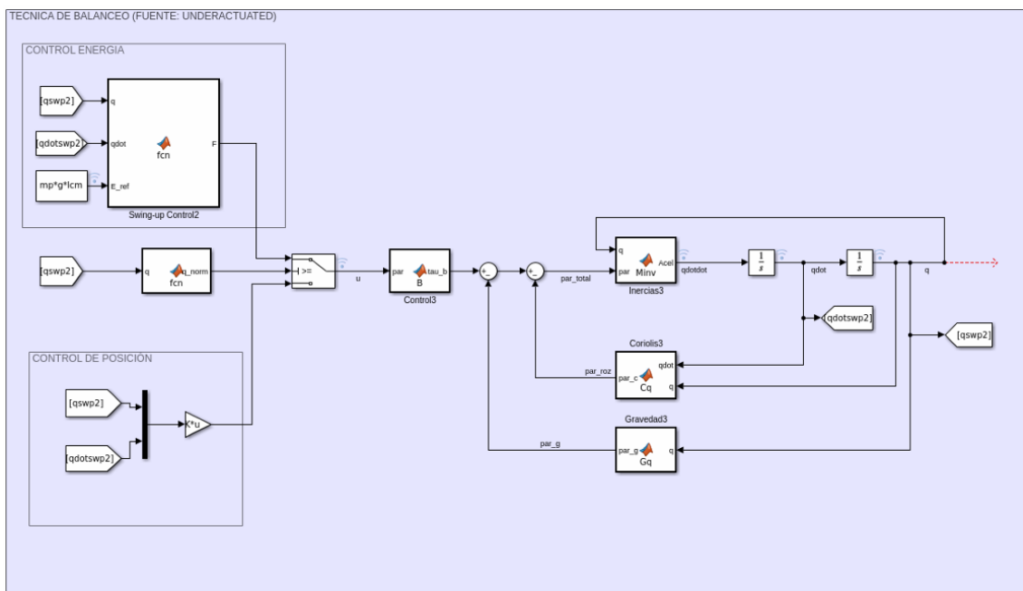
Figura 3.3: Diagrama de bloques conmutación entre controles
