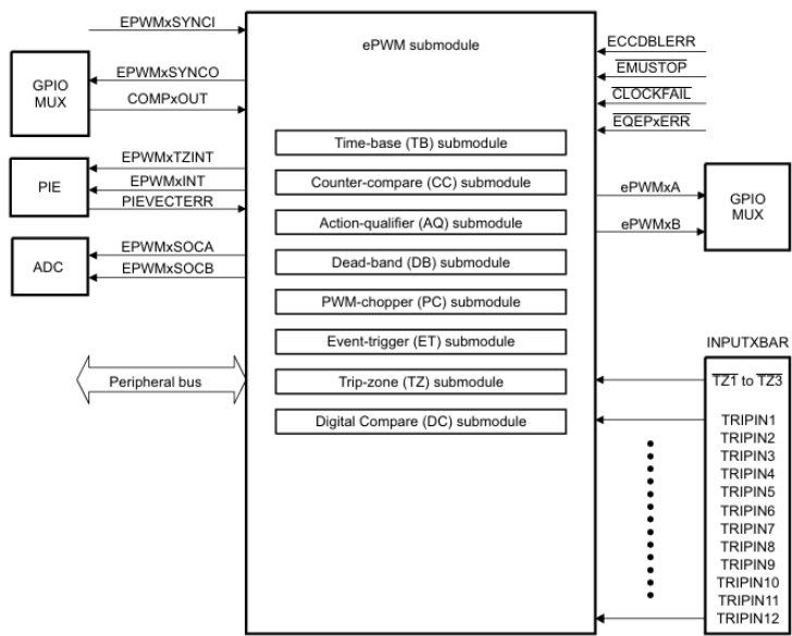
Figura 3.13: Diagrama de bloques y submódulos del periférico ePWM [22].
