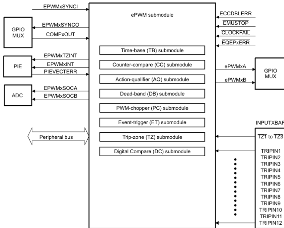
Figura 3.10: Diagrama de bloques y submódulos del periférico ePWM [22].
