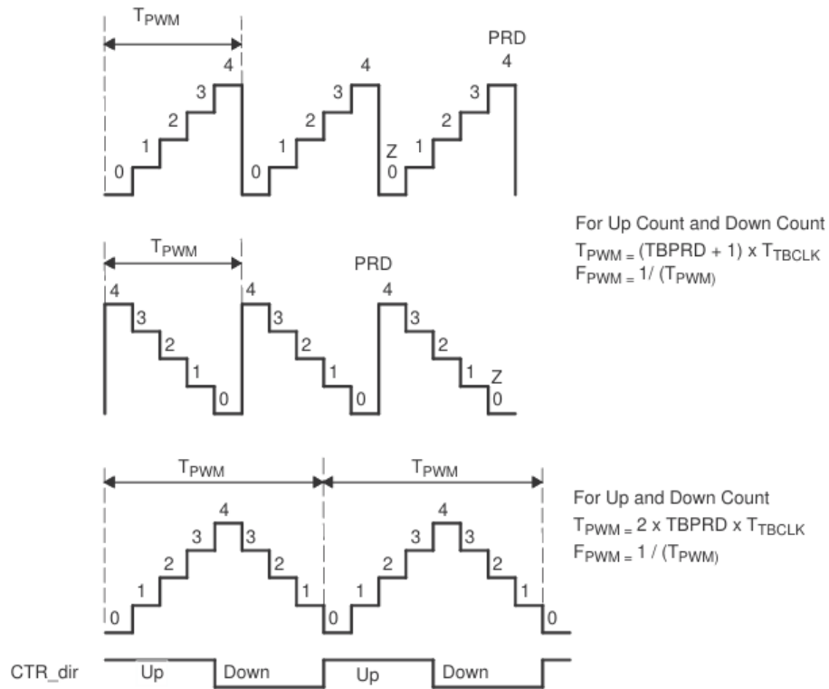
Figura 3.11: Modos de conteo del submódulo Time-base (TB) y ecuaciones de periodo [22].
