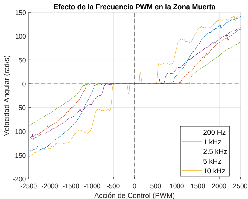
Figura 3.18: Efecto de la frecuencia de PWM en la zona muerta
