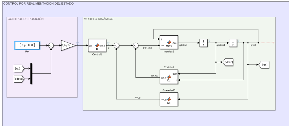
Figura 3.2: Diagrama de bloques con control de posición por realimentación del estado
