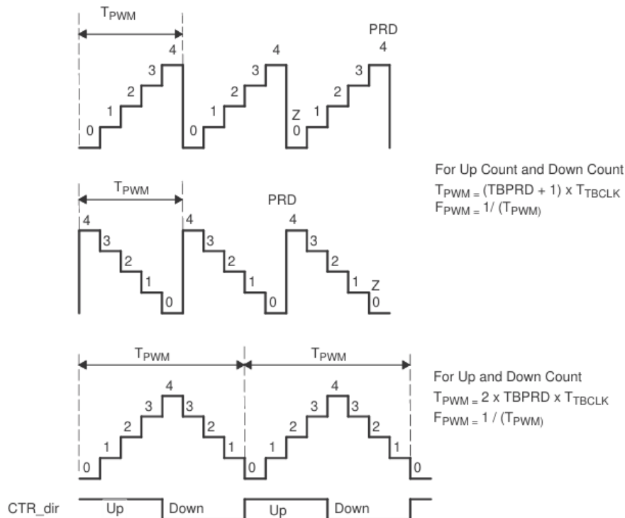
Figura 3.14: Modos de conteo del submódulo Time-base (TB) y ecuaciones de periodo [29].
