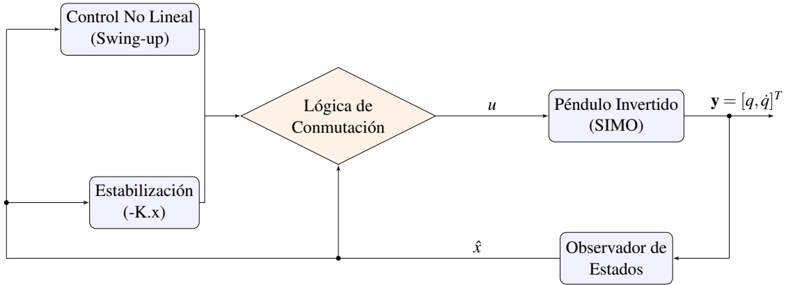
Figura 2.1: Arquitectura de control
