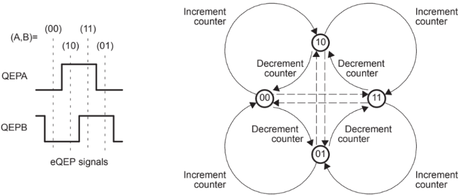
Figura 3.10: Máquina de estados, decodificación en cuadratura [22]
