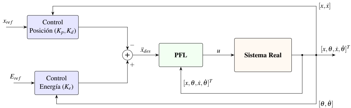
Figura 2.5: Diagrama de bloques Swing Up con control de posición
