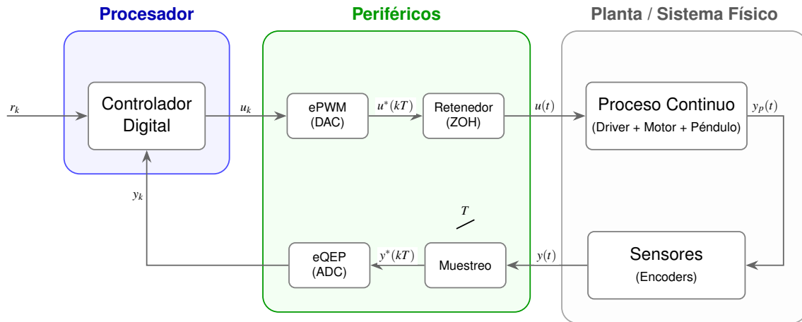
Figura 2.6: Arquitectura del sistema real
