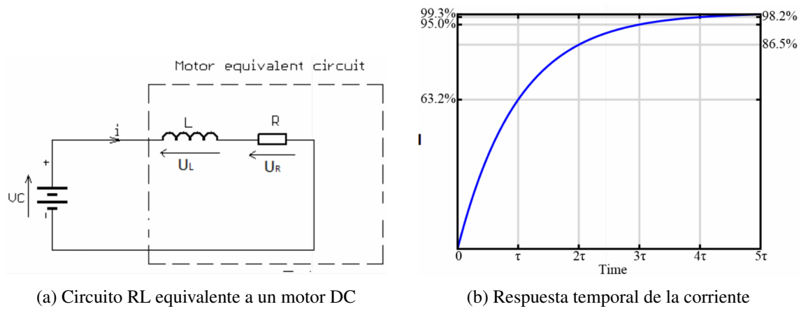
Figura 3.16: Circuito equivalente de un circuito motor DC y su dinámica ante entrada escalón
