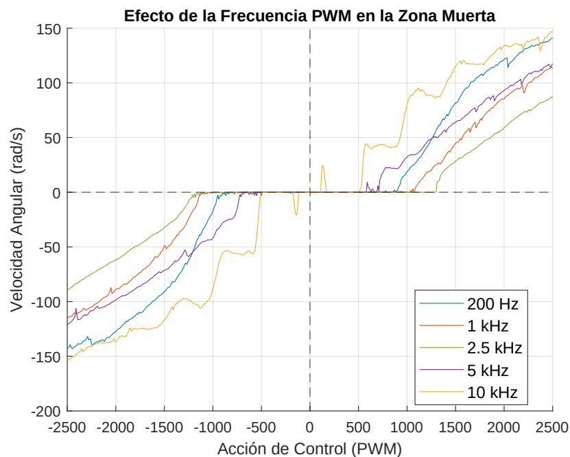
Figura 3.17: Efecto de la frecuencia de PWM en la zona muerta
