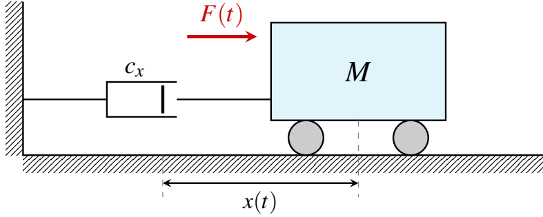
Figura 6.18: Modelo masa amortiguador
