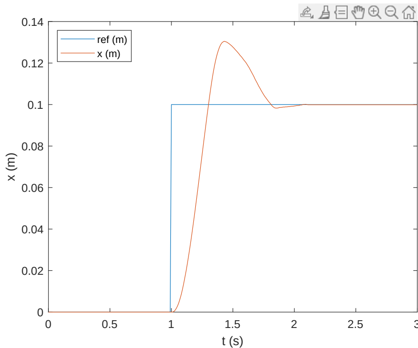
Figura 3.23: Dinámica M(s) obtenida experimentalmente
