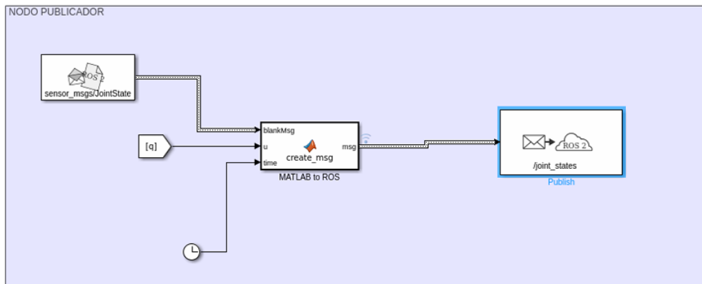
Figura 3.4: Arquitectura interna del nodo publicador en Simulink para la conversión y envío de datos a ROS
