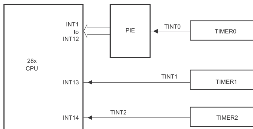
Figura 3.17: Rutas de las señales de interrupción asociadas a los TIMERS [22].
