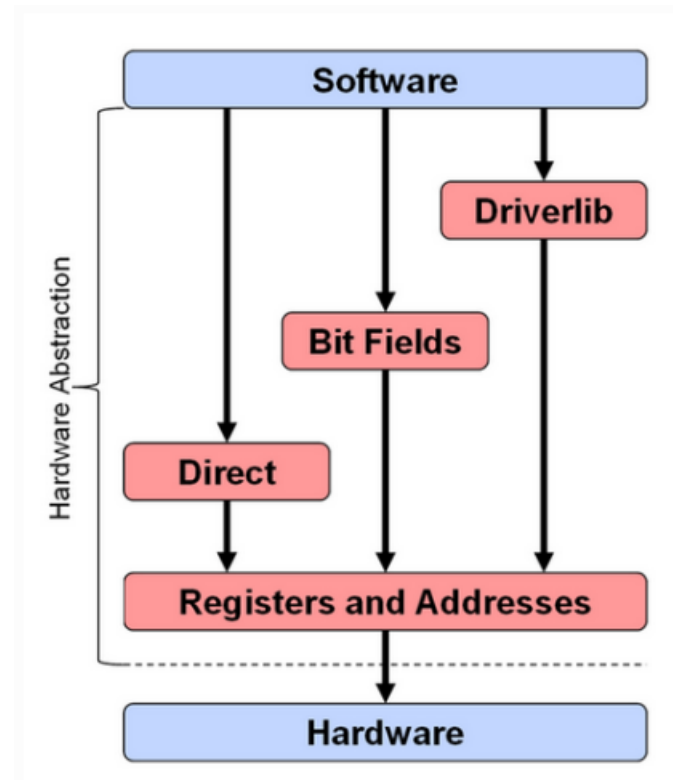
Figura 3.9: Niveles de abstracción para programar el microcontrolador [21]
