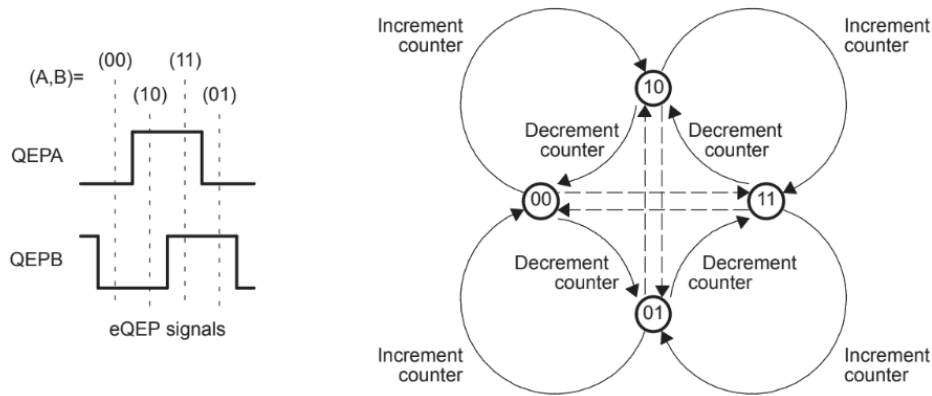
Figura 3.12: Máquina de estados, decodificación en cuadratura [22]
