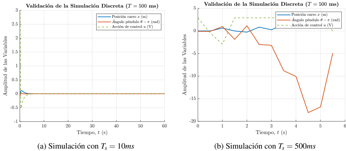
Figura 3.8: Dependencia de T_s en la simulación con expresiones recursivas
