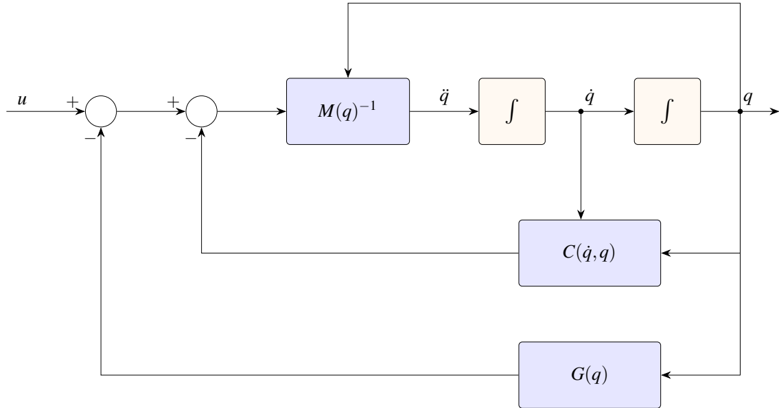
Figura 2.3: Diagrama de bloques del modelado
