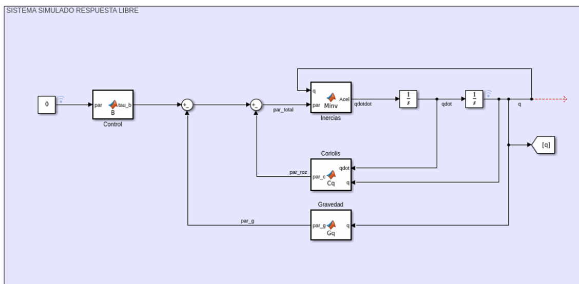
Figura 3.1: Arquitectura general del diagrama de bloques implementado en Simulink
