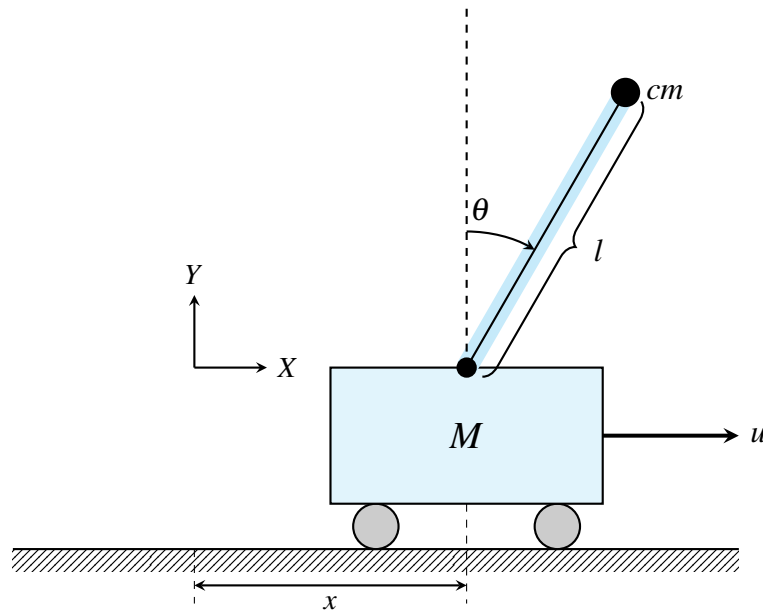
Figura 2.2: Esquema cinemático y convención de coordenadas del péndulo invertido sobre carro.
