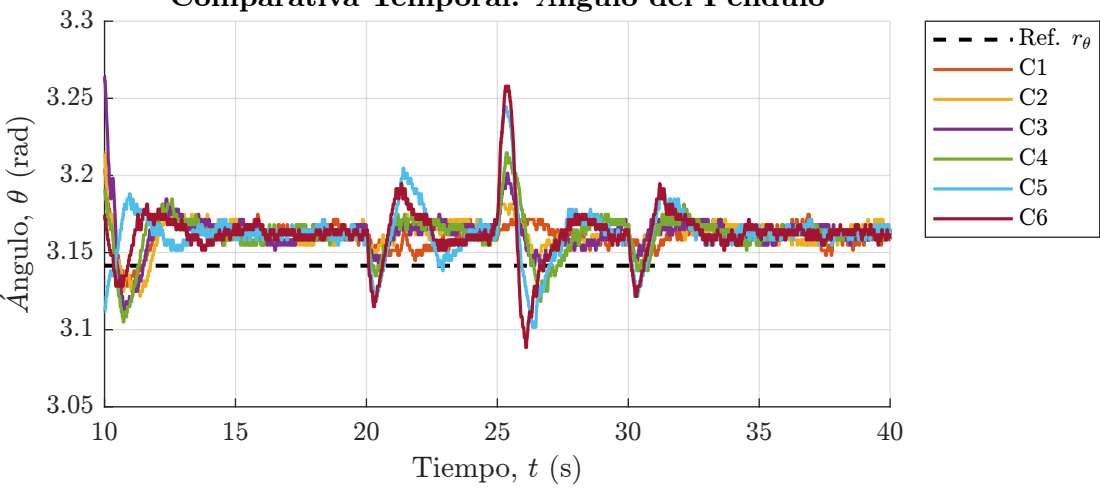
Comparativa Temporal: Ángulo del Péndulo
