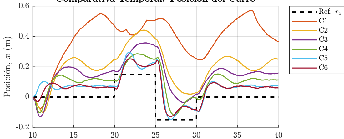
Comparativa Temporal: Posición del Carro
