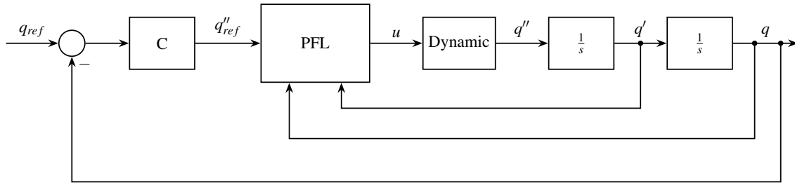
Figura 2.5: Diagrama de bloques técnica PFL
