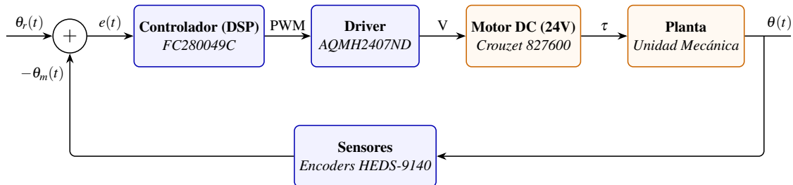
Figura 2.1: Arquitectura funcional del bucle de control cerrado para el péndulo invertido.
