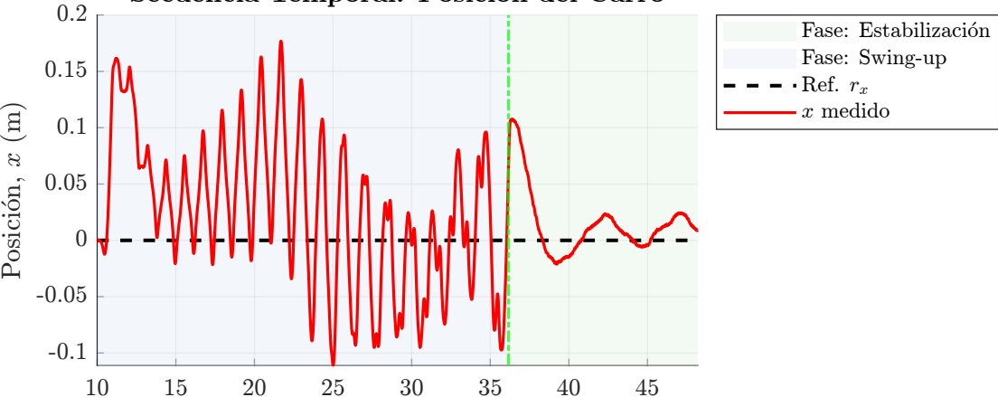
Secuencia Temporal: Posición del Carro
