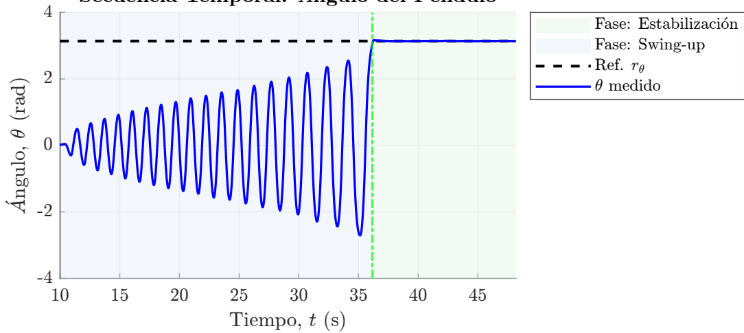
Secuencia Temporal: Ángulo del Péndulo
