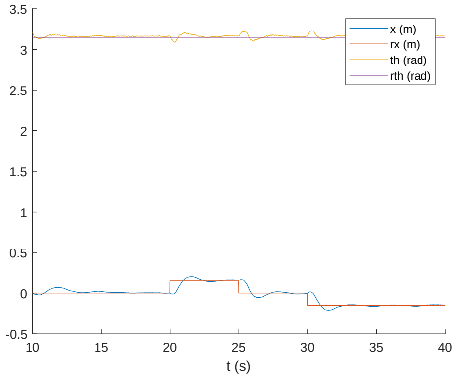
Figura 4.2: Control de posición con integrador sobre la planta real
