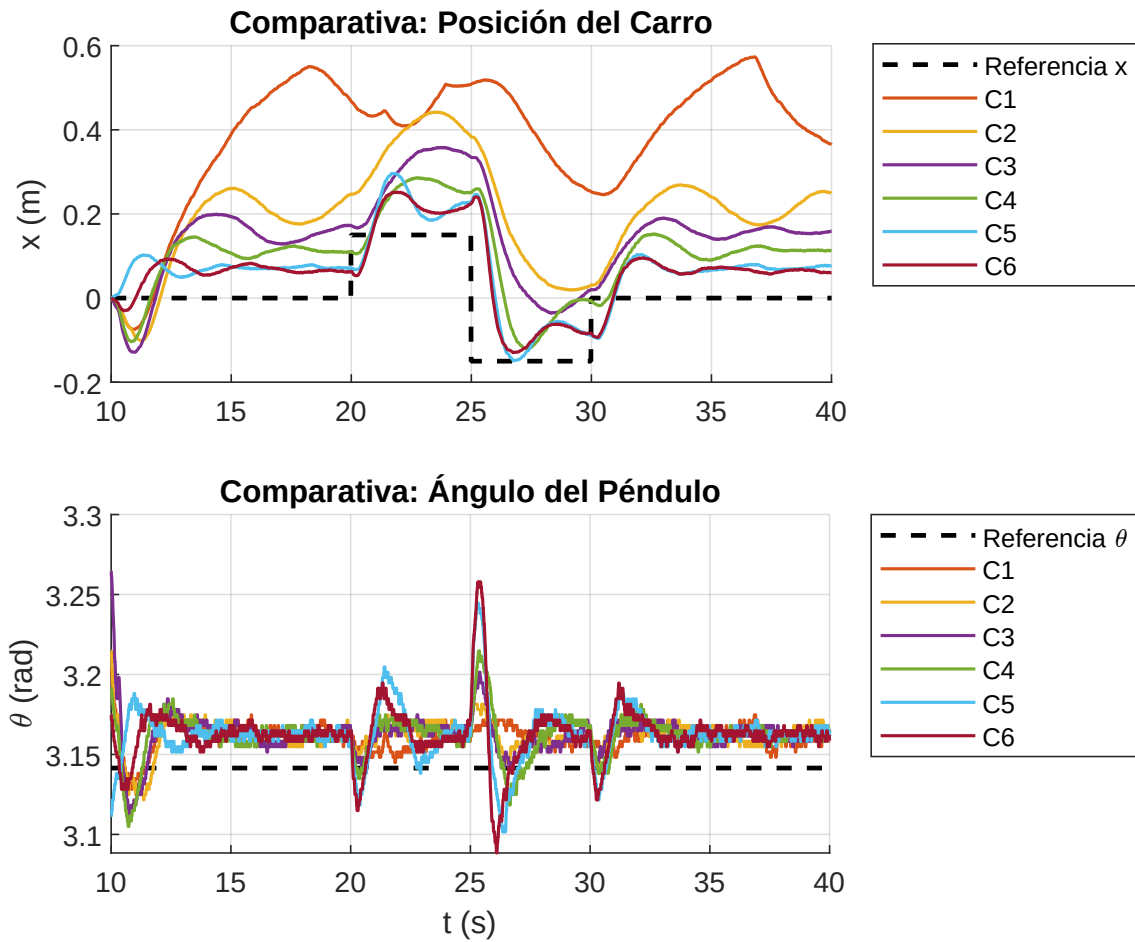
Figura 4.1: Desempeño de los controladores sobre la planta real
