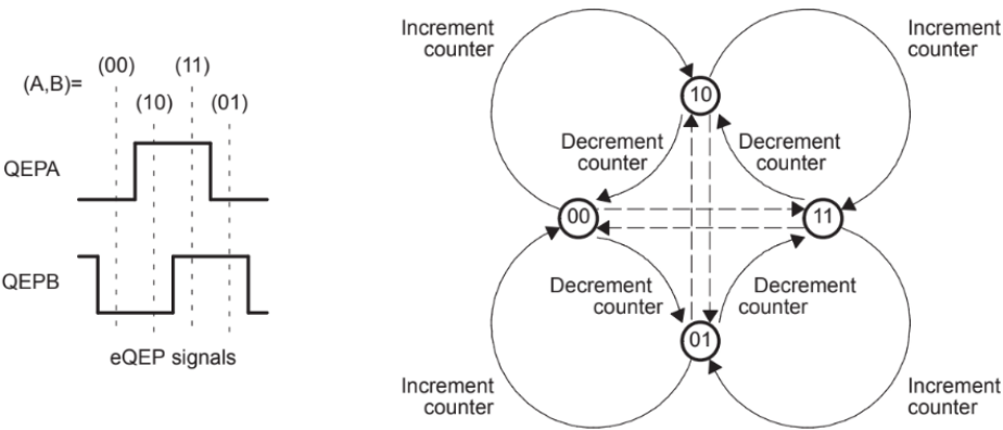
Figura 3.10: Máquina de estados, decodificación en cuadratura
