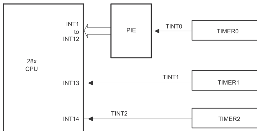
Figura 3.17: Rutas de las señales de interrupción asociadas a los TIMERS [29].
