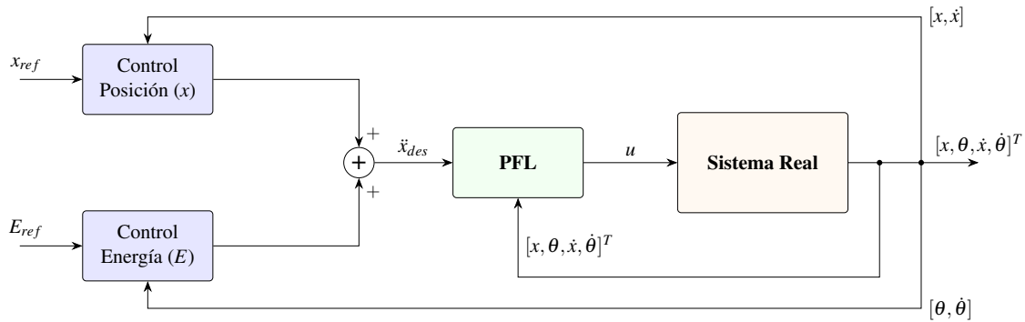
Figura 2.5: Diagrama de bloques técnica PFL
