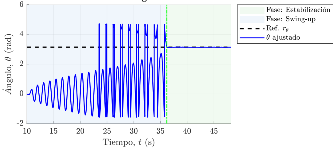
Secuencia Híbrida: Ángulo del Péndulo
