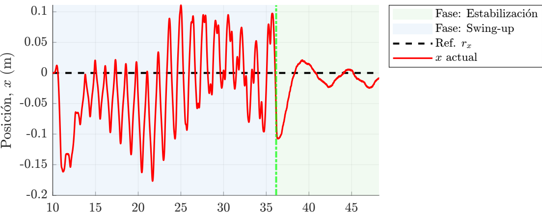
Secuencia Híbrida: Posición del Carro
