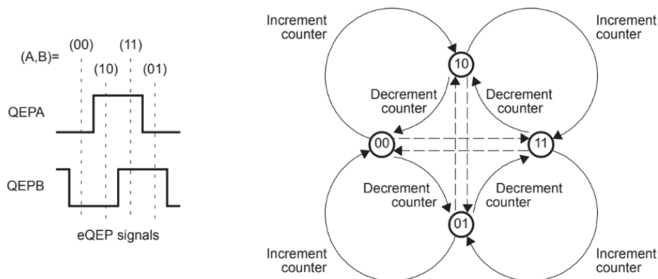
Figura 3.12: Máquina de estados, decodificación en cuadratura [33]
