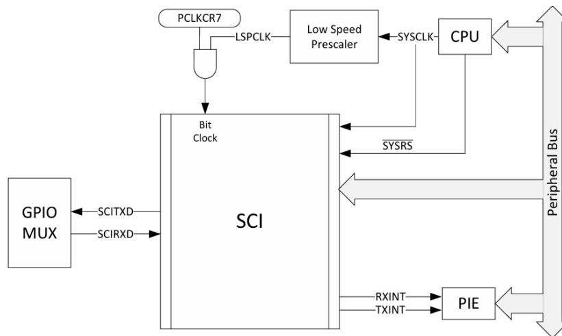
Figura 3.15: Diagrama de bloques y conexiones principales del periférico SCI [33]
