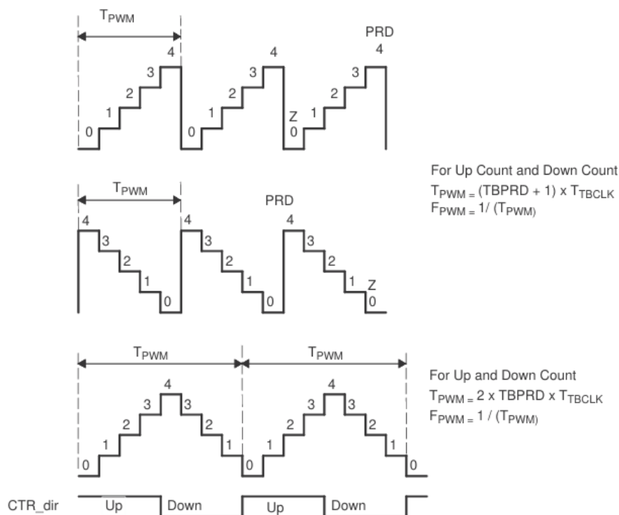
Figura 3.14: Modos de conteo del submódulo Time-base (TB) y ecuaciones de periodo [33].
