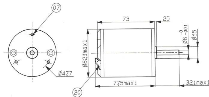
(a) Dimensiones del actuador [24]
