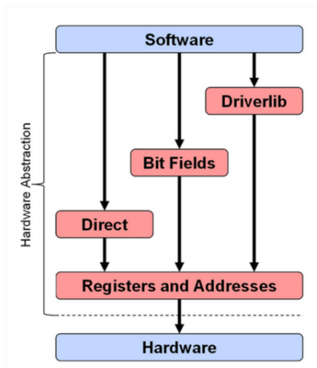
Figura 3.9: Niveles de abstracción para programar el microcontrolador [31]
