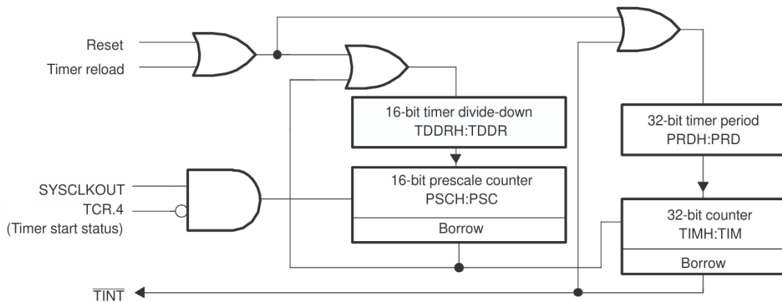
Figura 6.18: Diagrama lógico de bloques y registros asociados de los CPU Timers [33]
