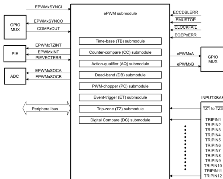
Figura 3.13: Diagrama de bloques y submódulos del periférico ePWM [33].
