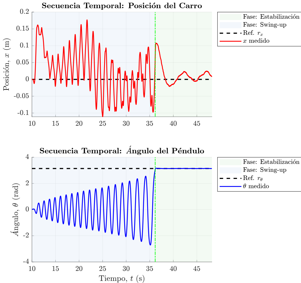
Figura 4.6: Control híbrido, conmutación entre Swing-up y control de posición
