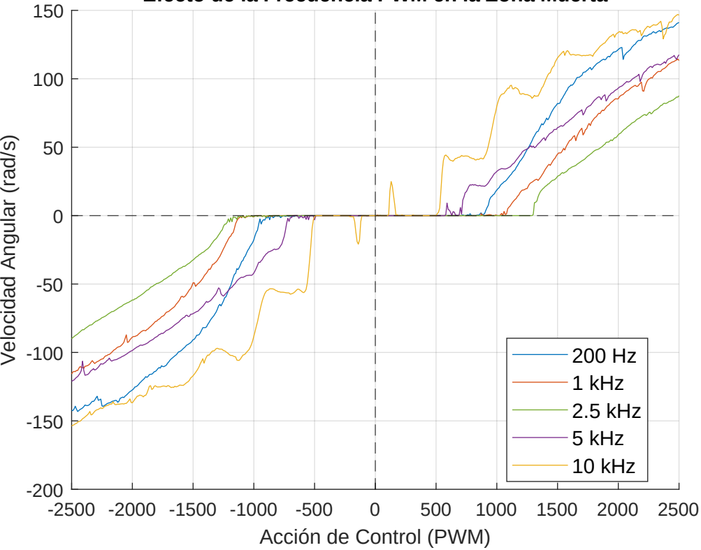
Efecto de la Frecuencia PWM en la Zona Muerta
