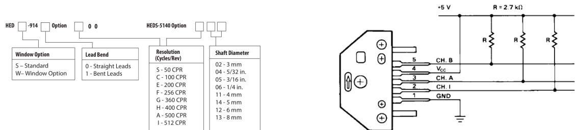
(a) Especificaciones módulo de detección y disco óptico según modelo específico
