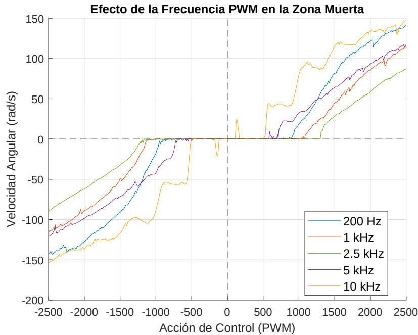
Figura 3.15: Efecto de la frecuencia de PWM en la zona muerta
