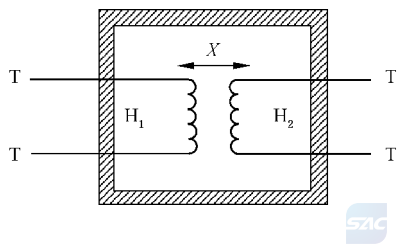
图 D.3 两个危险带电电路的外部可触及端子的防护
