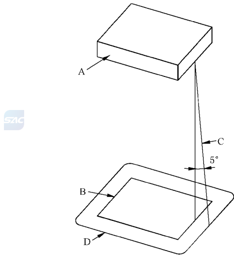
图 5 挡板
