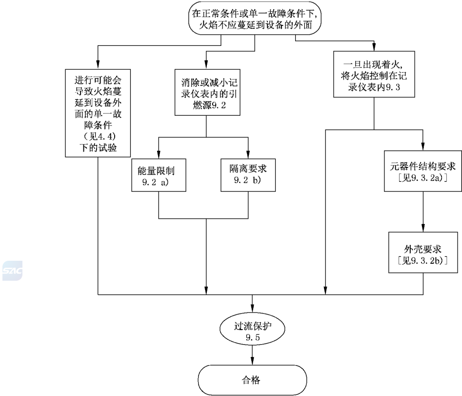
图 4 说明防止火焰蔓延要求的流程图
